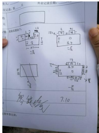
房屋平面草图绘制
